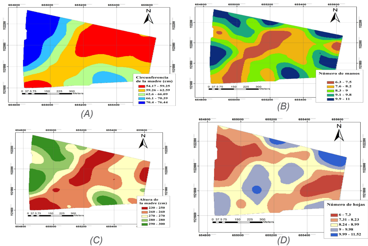
Figura 9. Distribución espacial de las variables morfométricas aéreas de las plantas de banano: (A) circunferencia de la madre, (B) número de manos, (C) altura de la madre y (D) número de hojas. Fuente: elaboración propia.
