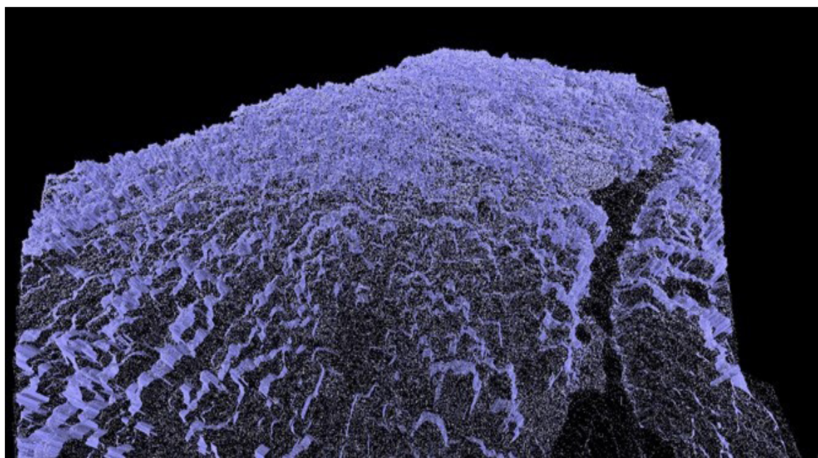
Figura 7. Malla TIN
