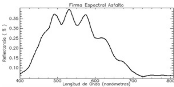
Figura 13. Firma espectral de asfalto representada en niveles de reflectancia y longitud de onda en nanómetros Fuente: elaboración propia.
